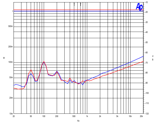
Übersprechdämpfung L/ R // R/ L 1 kHz/ typ. \geq 80\text{dB} (-86,83 dB/ -86,92 dB)
