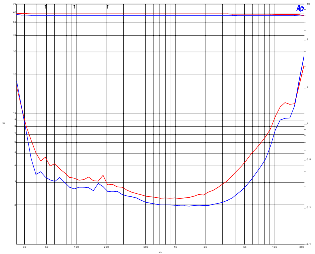
Verzerrungen THD+N 2x 60 Watt/ Sinus 1kHz / typ. \leq 1\% (0,24% / 0,208%) SEL-Version
