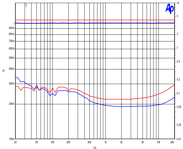
Verzerrungen THD+N 2 x 1 Watt / Sinus 1kHz / typ. \leq 0,1\% (0,055% / 0,075%)
