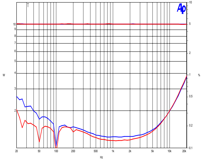
Verzerrungen THD+N 2x 10 Watt /Sinus 1 kHz / typ. \leq 0,3\% (0,142% / 0,126%)
