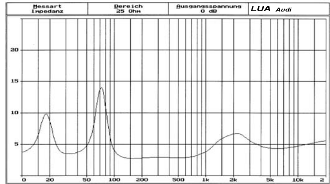
Lautsprecher: Impedanzkurve
