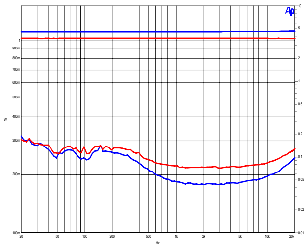
Distortions THD+N 2x 1 Watt / Sine 1kHz / typ. \leq 0,1\% (0,047% / 0,076%)
